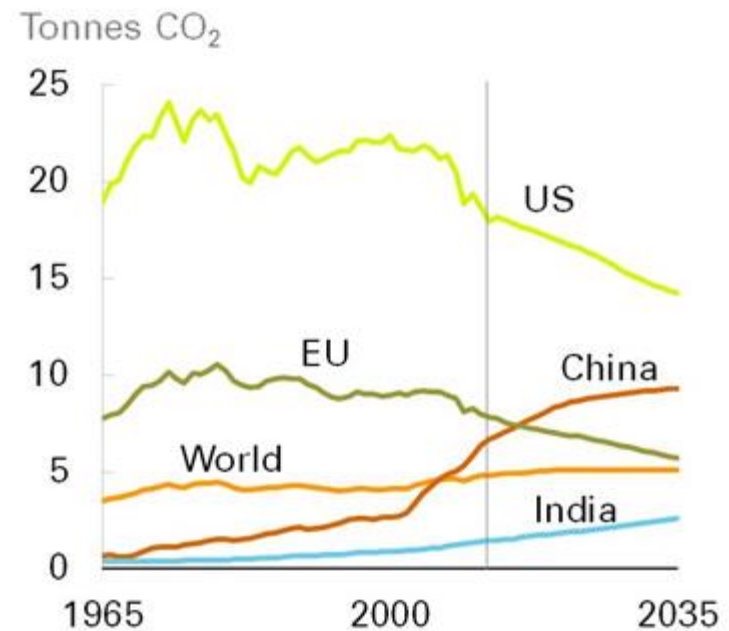
Emissions per capita
